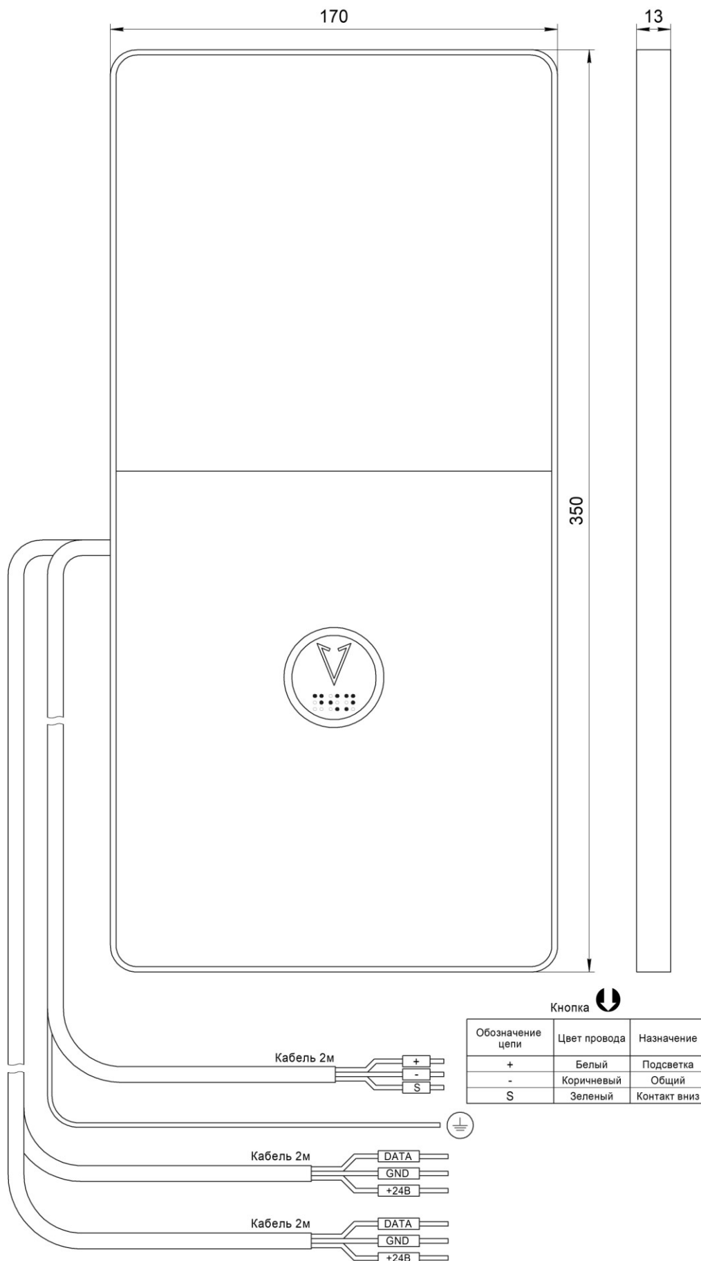
Рис.1 Внешний вид, габаритные и установочные размеры Вызывного поста МАЛАХИТ НШЕК.468381.076-01
